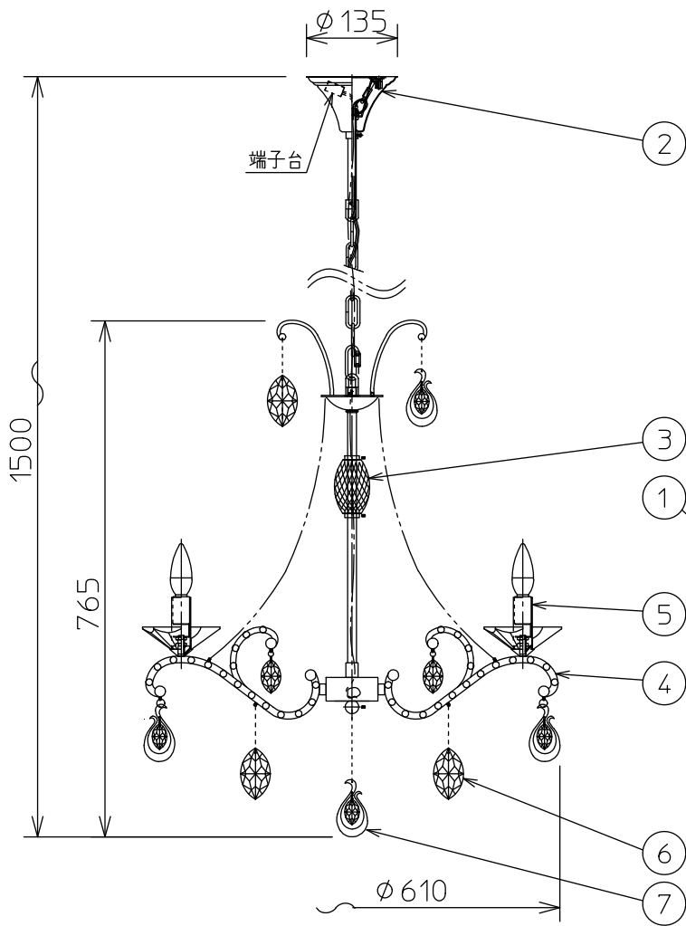
灯具配置図
