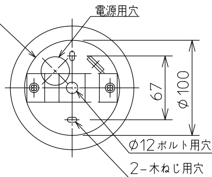
取付部詳細
