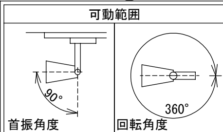
取付部
