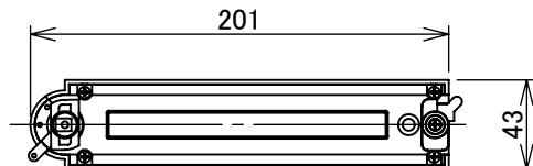
取付部
