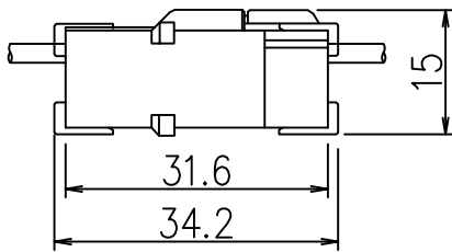
コネクタ接続時 外形寸法
