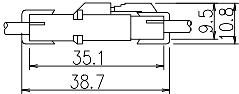
コネクタ接続時 外形寸法
