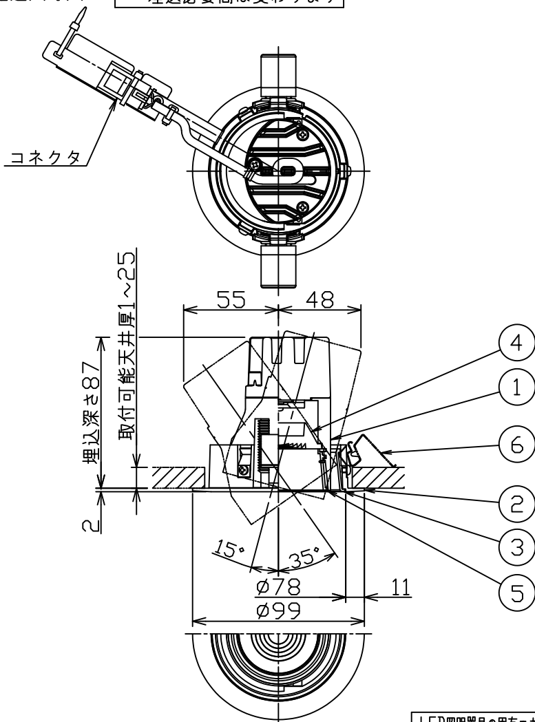
埋込穴寸法
