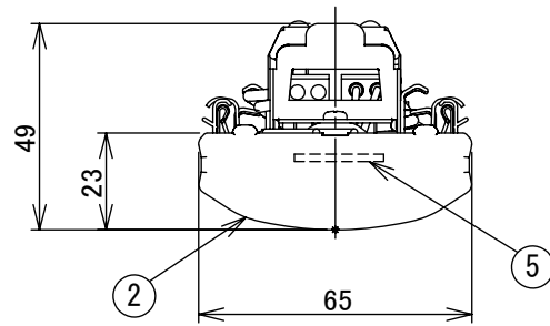
側面詳細図
