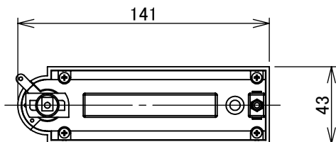
取付部
