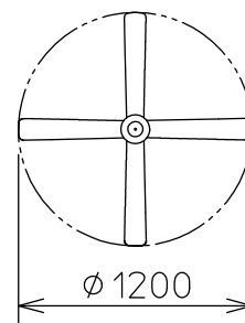
羽根配置図
