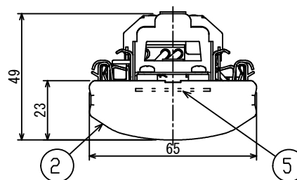
側面詳細図
