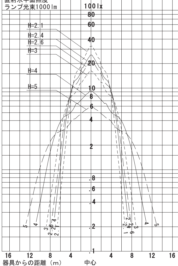
配光曲線 ランプ光束1000lm
