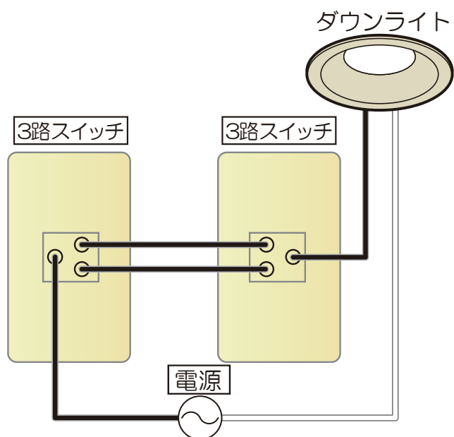
[3路スイッチ配線]
