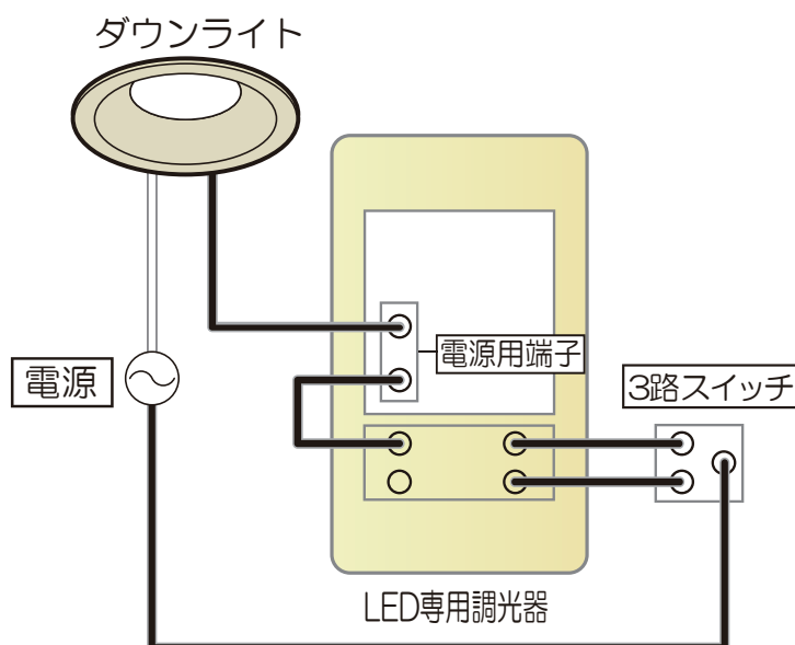
[3路スイッチ配線]
