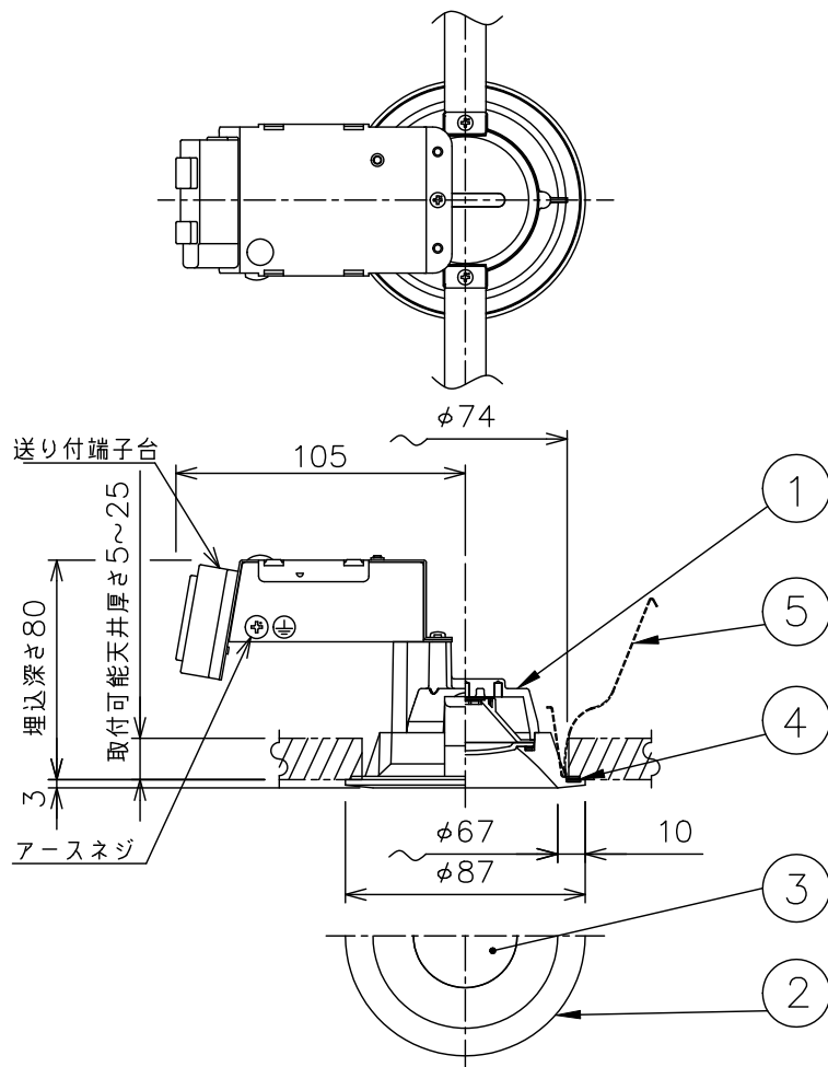
埋込穴寸法
