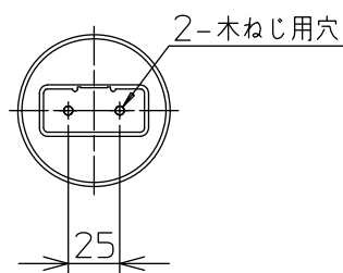
取付部詳細
