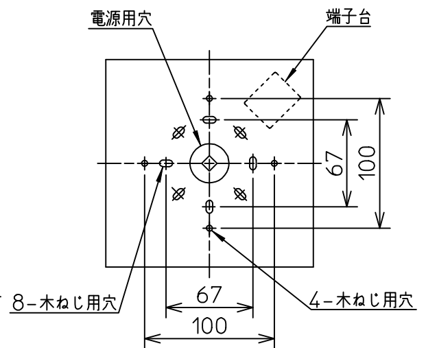
取付部詳細
