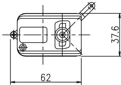
取付部詳細
