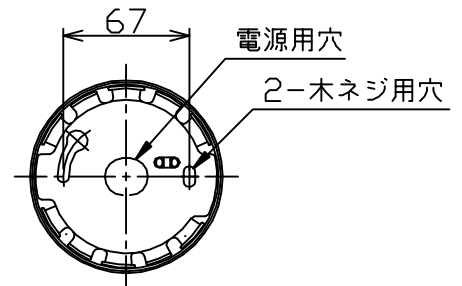
取付部詳細
