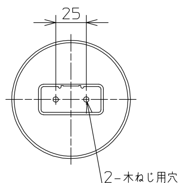
取付部詳細
