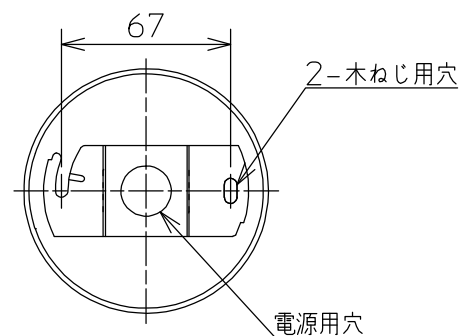
取付部詳細
