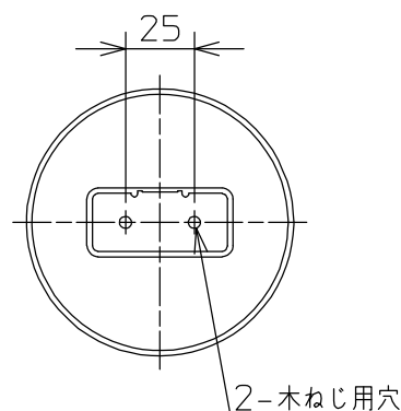
取付部詳細
