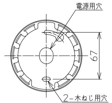
取付部詳細
