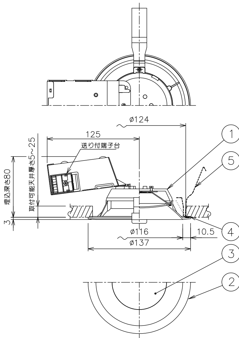
埋込穴寸法
