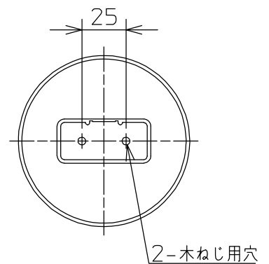
取付部詳細
