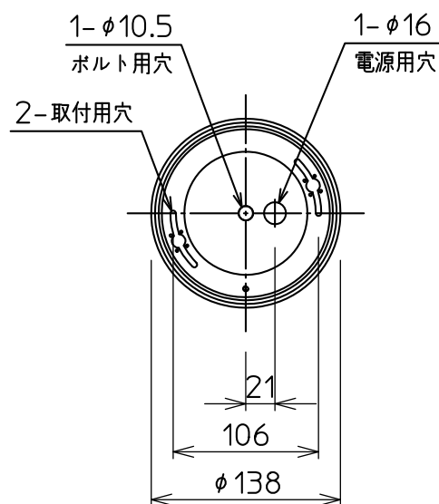
取付部詳細
