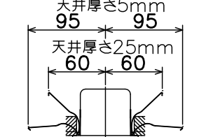
パネの広がり寸法
