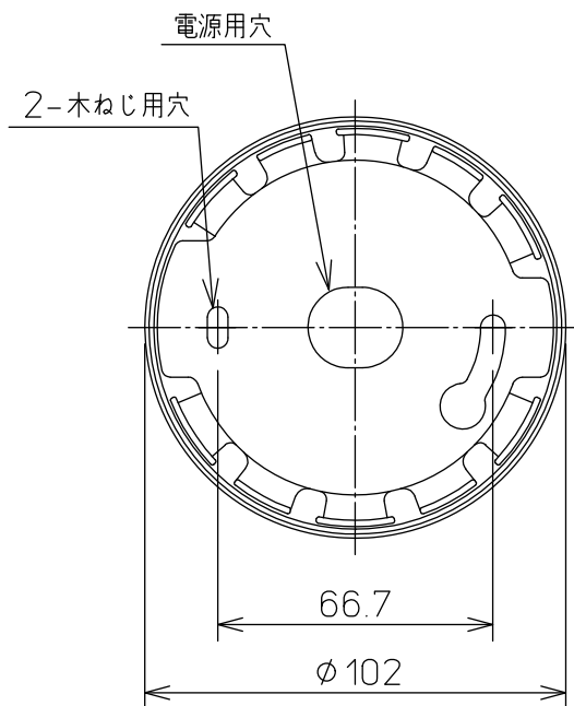
取付部詳細
