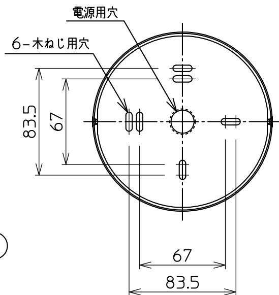
取付部詳細
