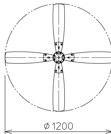
羽根配置図
