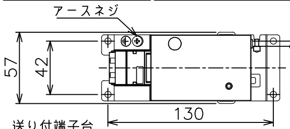
埋込穴寸法
