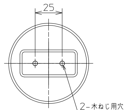
取付部詳細
