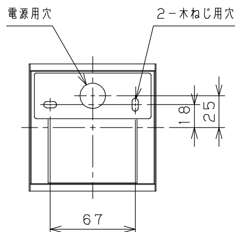
取付部
