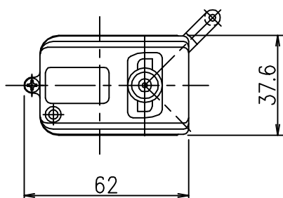
取付部詳細
