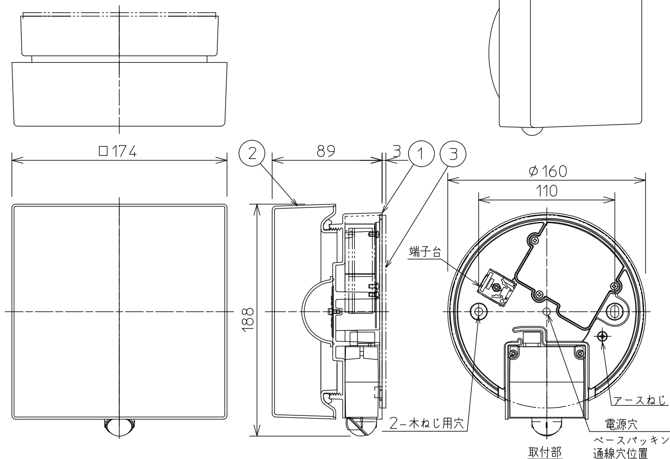
姿図
