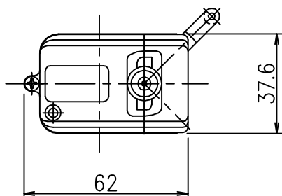
取付部詳細
