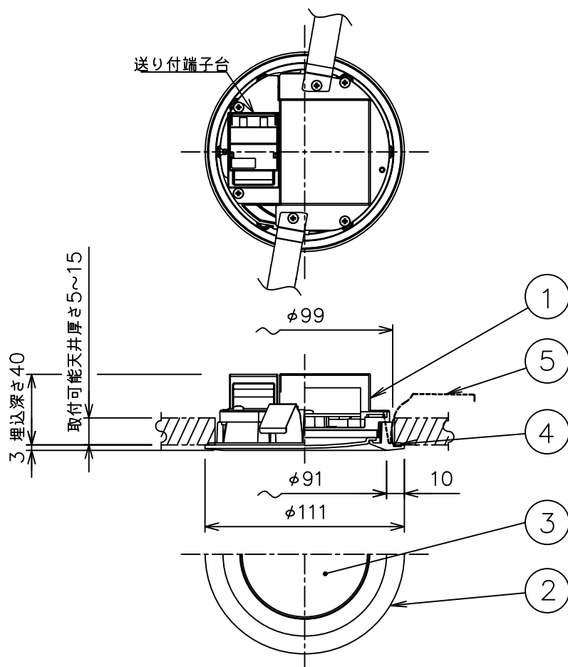
埋込穴寸法
