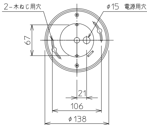
取付部詳細
