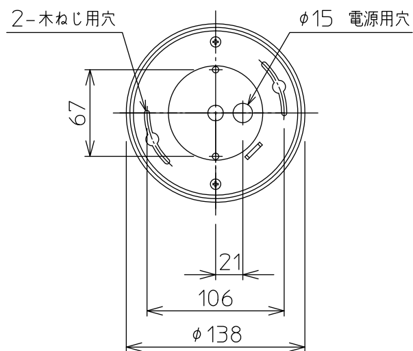
取付部詳細
