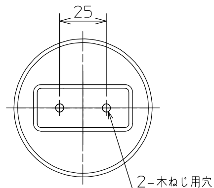
取付部詳細
