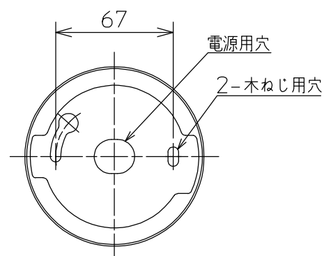
取付部詳細
