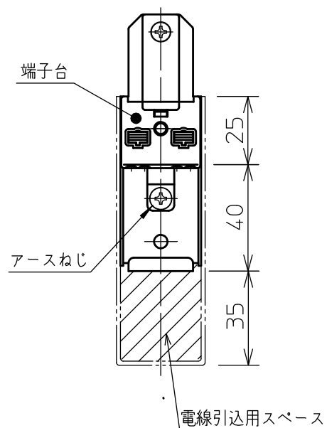
端子台詳細
