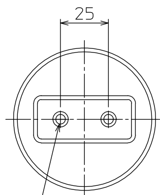
取付部詳細
