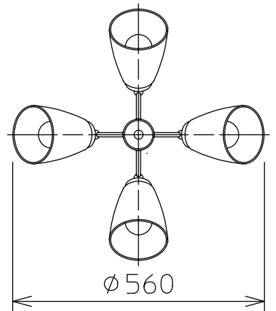
灯具配置図
