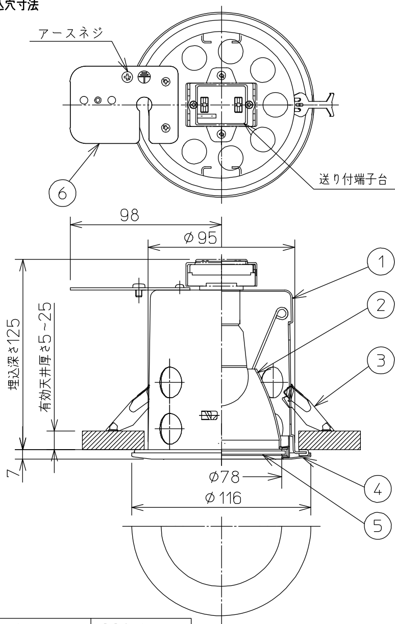
埋込穴寸法
