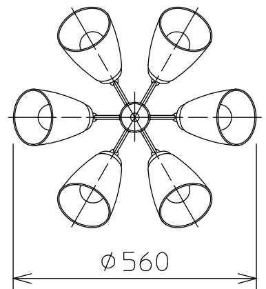
灯具配置図
