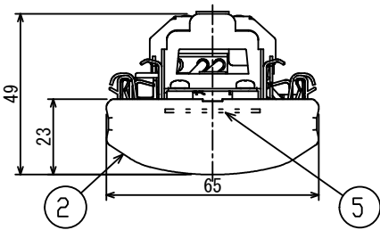
側面詳細図
