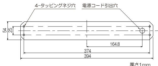
パッキン寸法
