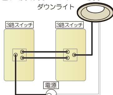
〔3路スイッチ配線〕
