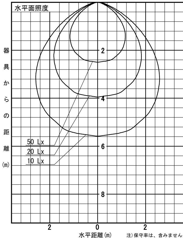
配光曲線
