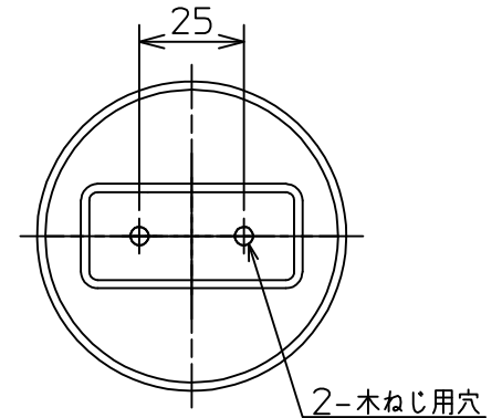
取付部詳細
