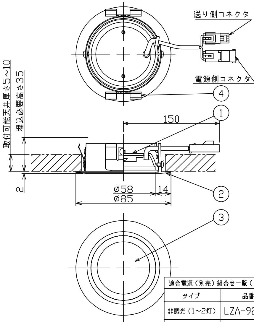
埋込穴寸法
